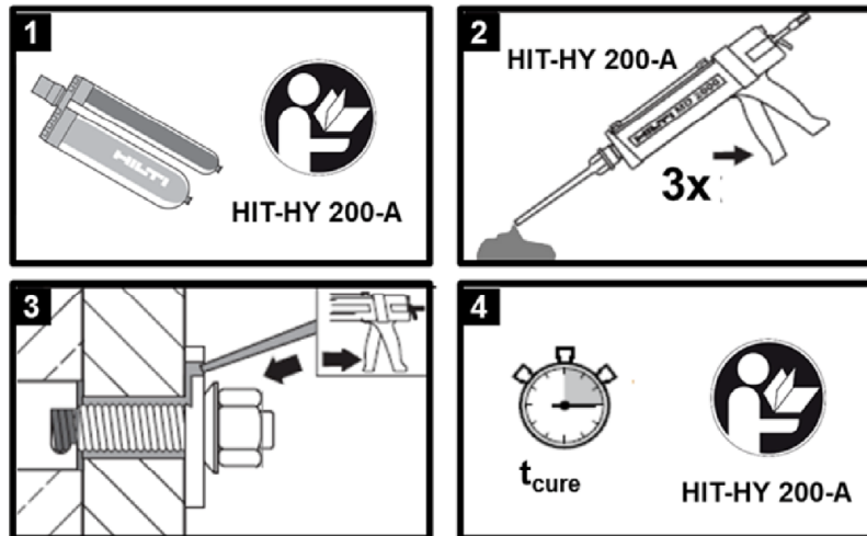
Bild 15: Montageanweisung: Verfüllung mit Injektionsmörtel Hilti HIT-HY 200-A (optional)
