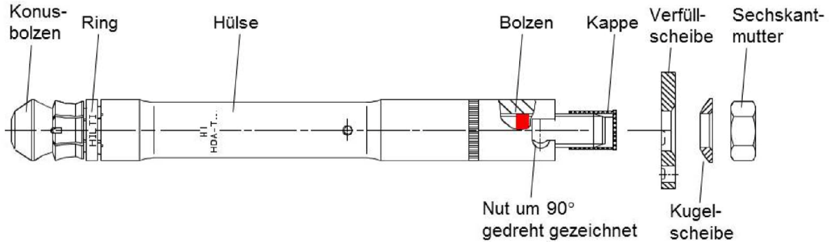
Bild 3: Durchsteckdübel HDA-T(R)
