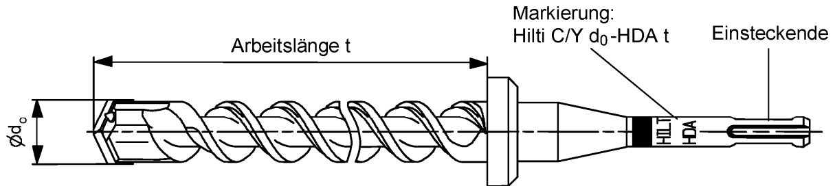
Bild 11: Bundbohrer HDA-B
