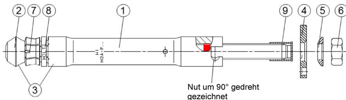
Bild 7: Durchsteckdübel HDA-T / HDA-TR
