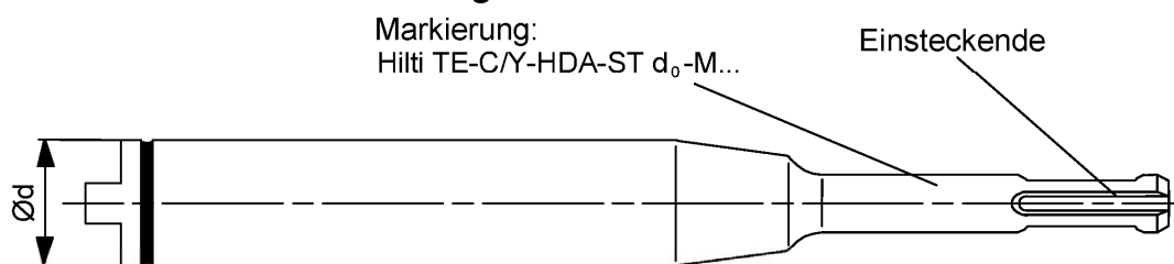
Bild 12: Setzwerkzeug HDA-ST
