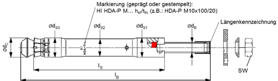
Bild 8: Vorsteckdübel HDA-P(R)
