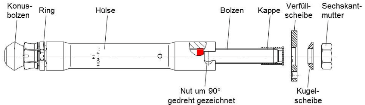
Bild 1: Vorsteckdübel HDA-P(R)
