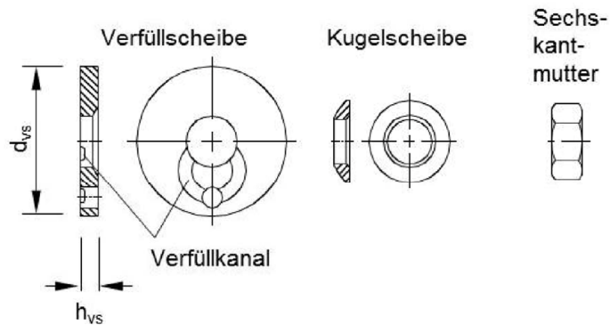
Bild 10: Verfüll-Set
